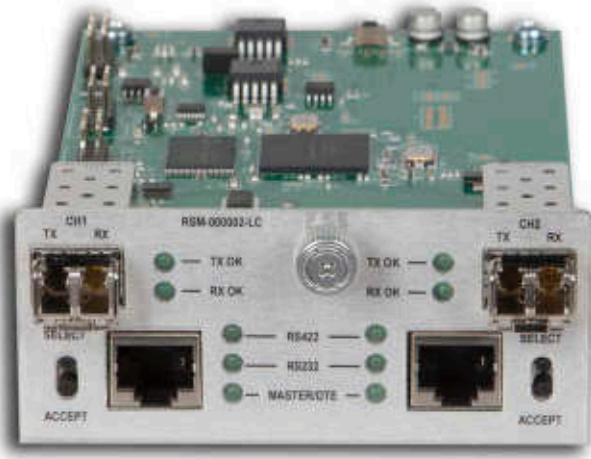
RS-232/422 Extender Module
